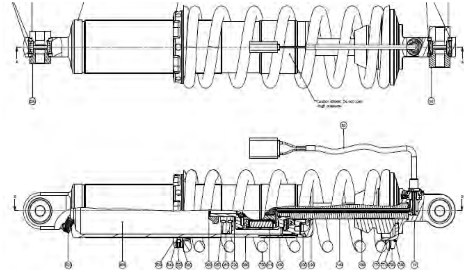
Schema-Zeichnung eines elektronischen Federbeins
